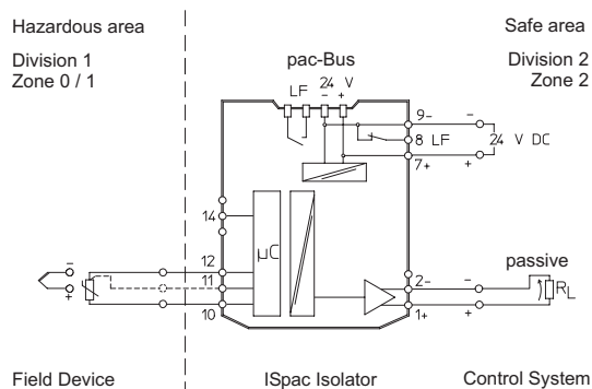
Esquema de conexiones 9182/10-51-11; 9182/10-51-13
