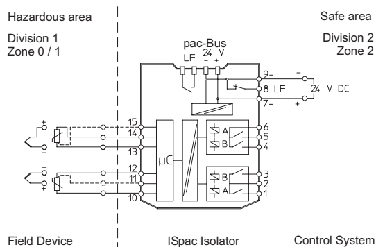
Esquema de conexiones 9182/20-50-12
