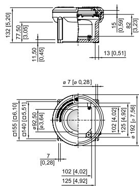
Tamaño de envolvente 2 con ventana
