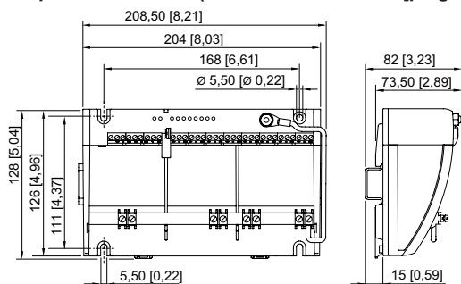
Acoplamiento de dispositivo de campo, 8 pistas, sin envolvente
