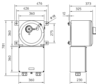
Esquema de medida (todas las medidas en [pulgadas]) – Se reserva el derecho a modificaciones
