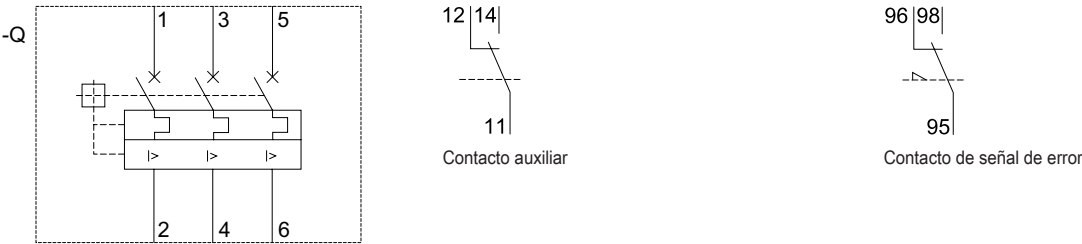
Diagrama unifilar del dispositivo
