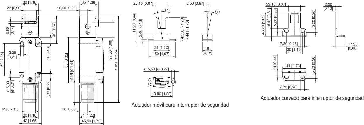
Interrupor de seguridad 8070/2-.-AZ-U50
