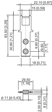
Actuador para interrupor de seguridad recto
