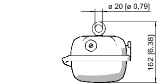
Tornillo de cáncamo montado en tuerca autoinsertable de la luminaria
