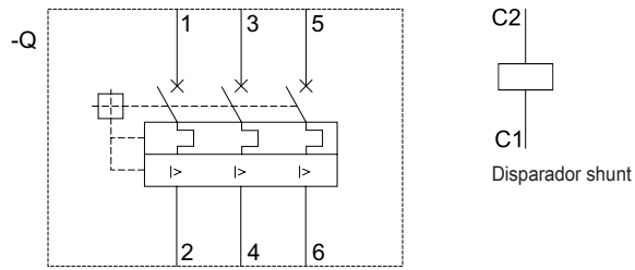
Diagrama unifilar del dispositivo
