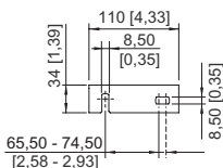
Escuadra de fijación de pared montada en riel de montaje DIN
