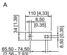
Escuadra de fijación de pared montada en raíl de montaje DIN
