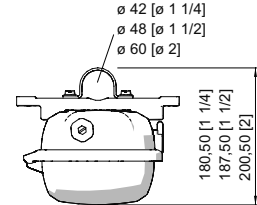
Abrazadera de tubo montada en raíl de montaje DIN
