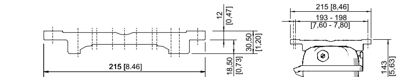
Raíl de montaje DIN
