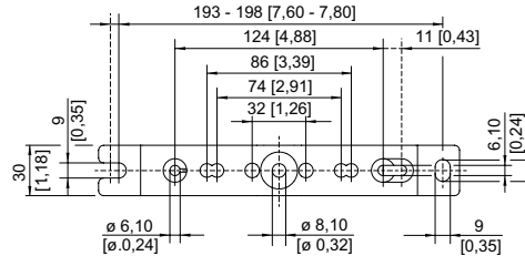
Rail de montaje DIN
