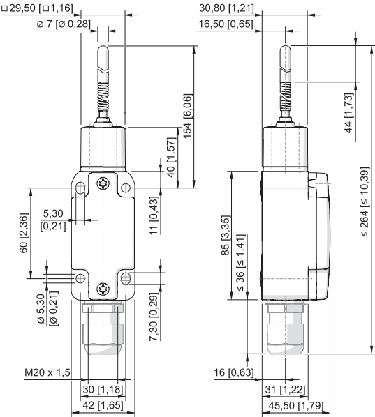
Varilla elástica 8070/2--TK-U60
