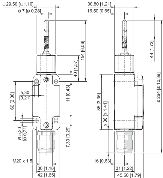
Varilla elástica 8070/2--TK-U60
